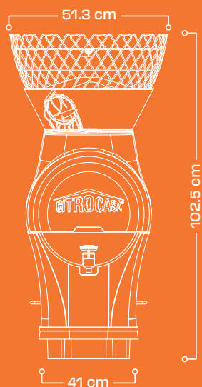
Vorderansicht
