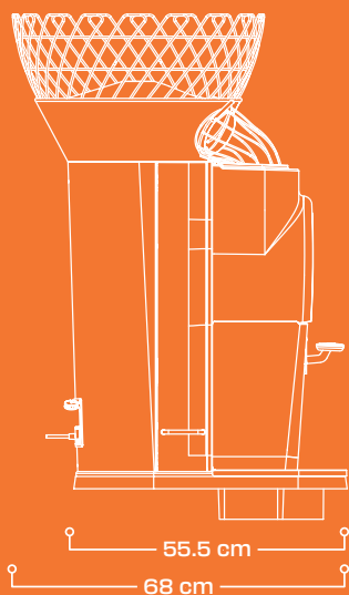
Seitenansicht
