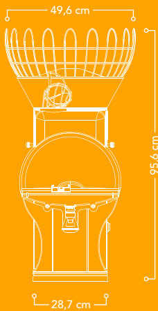
Vorderansicht
