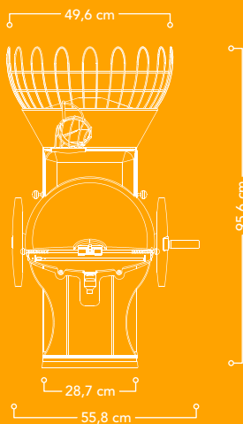
Vorderansicht
