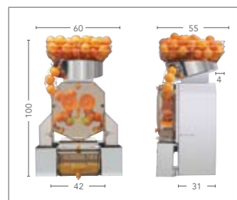
Citrocasa 8000 XB mit Juice-Tank Art.-Nr. 80.002
