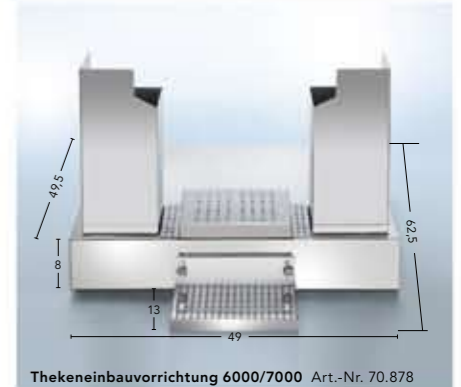
Thekeneinbauvorrichtung 6000/7000 Art.-Nr. 70.878
