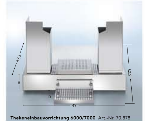
Thekeneinbauvorrichtung 6000/7000 Art.-Nr. 70.878
